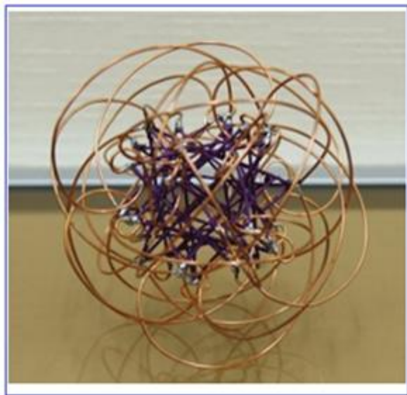
Рис. 1.1. Внешний звездчатый триандазиоэдр
