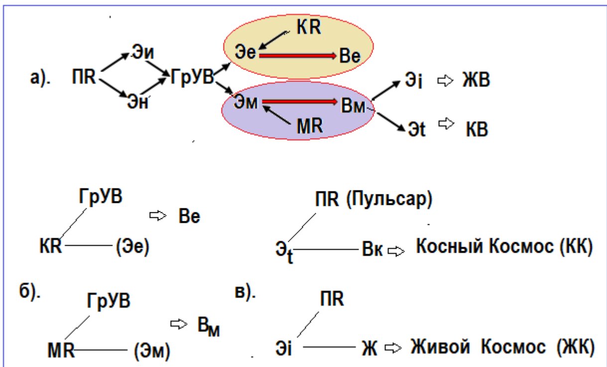
Рис. 2. Формирование живого (ЖВ) и косного (КВ) вещества
