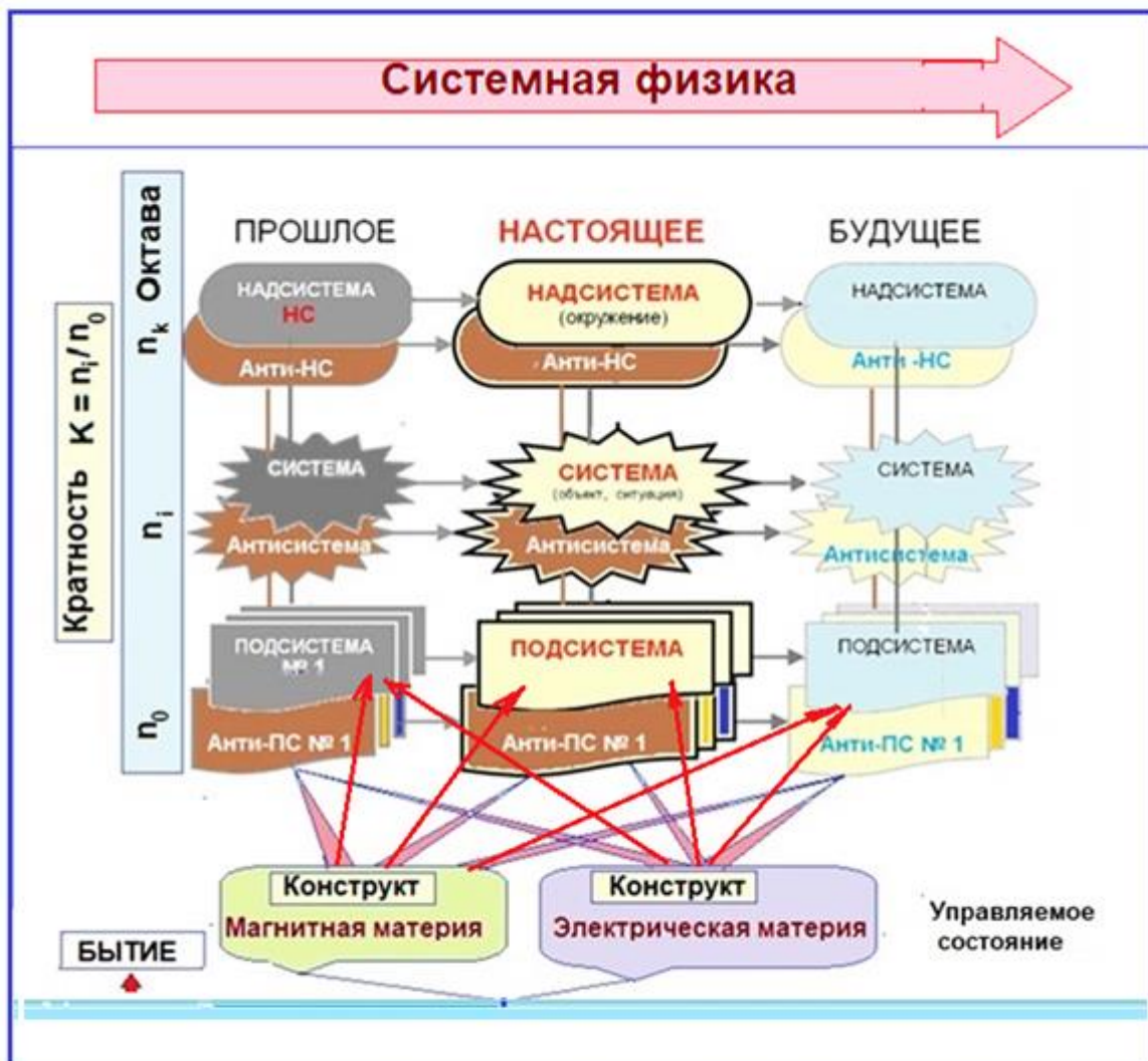
Схема многоэкранного мышления: этапы развития вещества на уровне конструктов разной масштабной мерности во времени.
