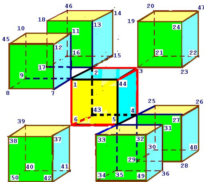
Кубическая решётка золота
