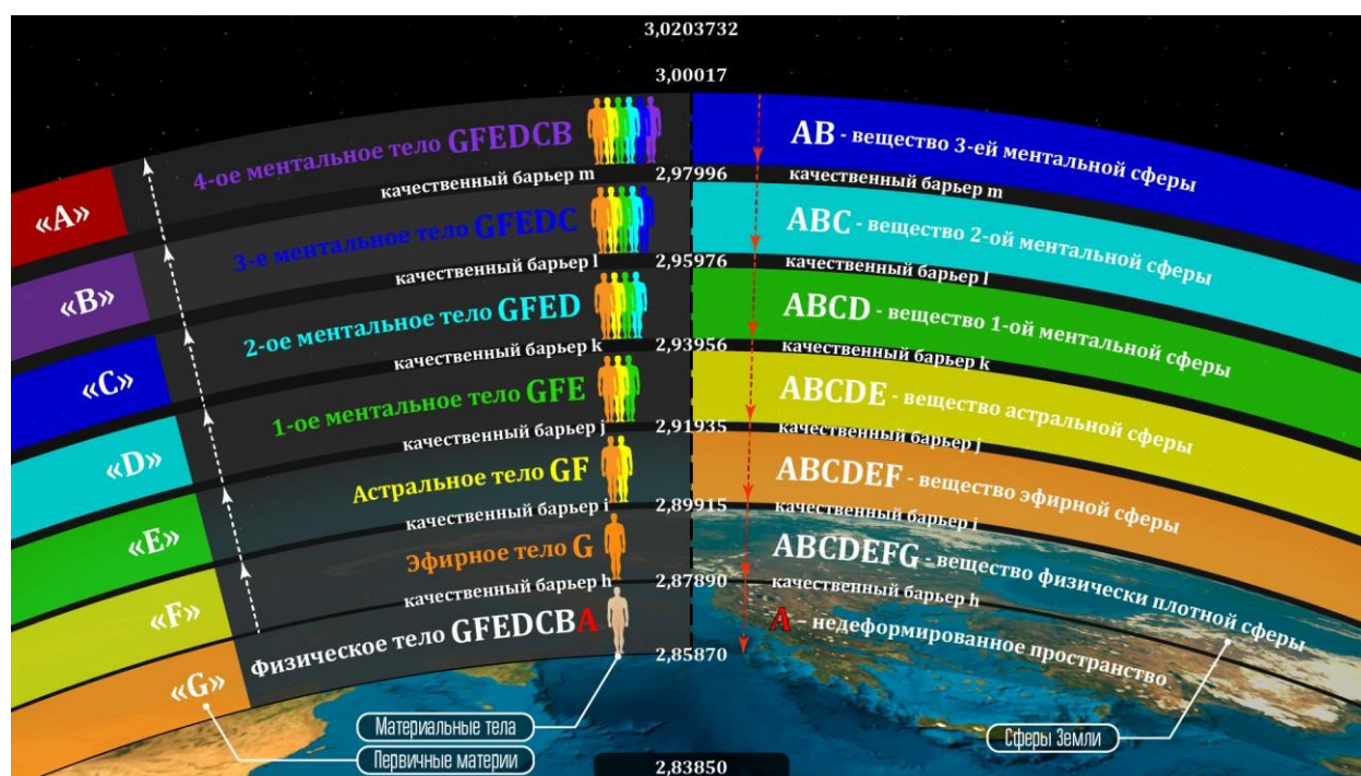
Рис. 3 Сводная схема соотношения мерностей первичных и гибридных материй, материальных тел человека.
